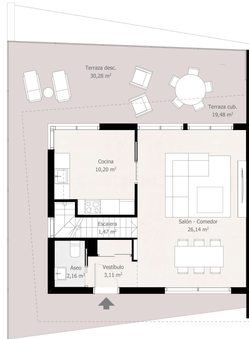
Planta acceso. Opción cocina cerrada
